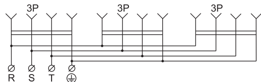
3x3P+PE
