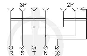
3P+PE/2P+PE
