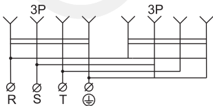
3P+PE/2P+PE
