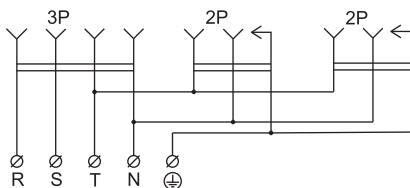
3P+PE/2x2P+PE
