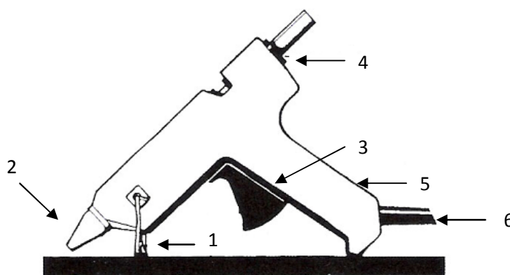
Рис. 1. Пістолет термоклейовий COMPASS GG188AA.
